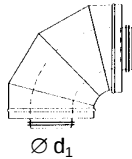
Bogen BUI 90°
